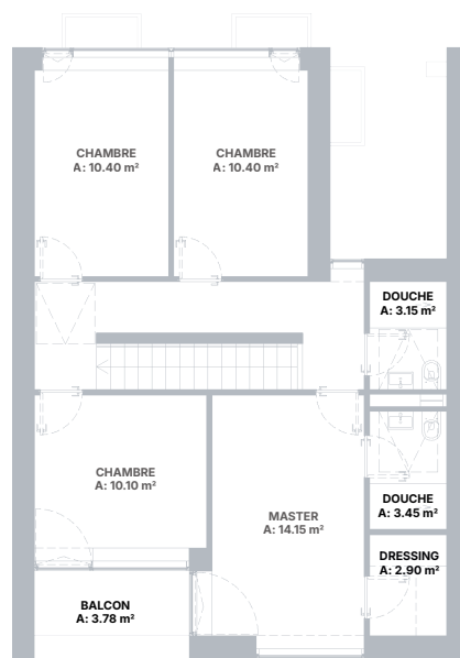
Étage
