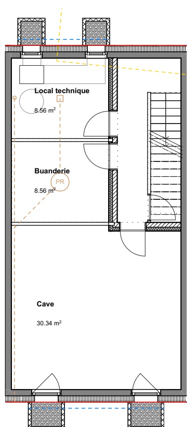
Sous-sol
